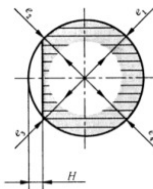
图 B.2 淬透深度的测定示意图
