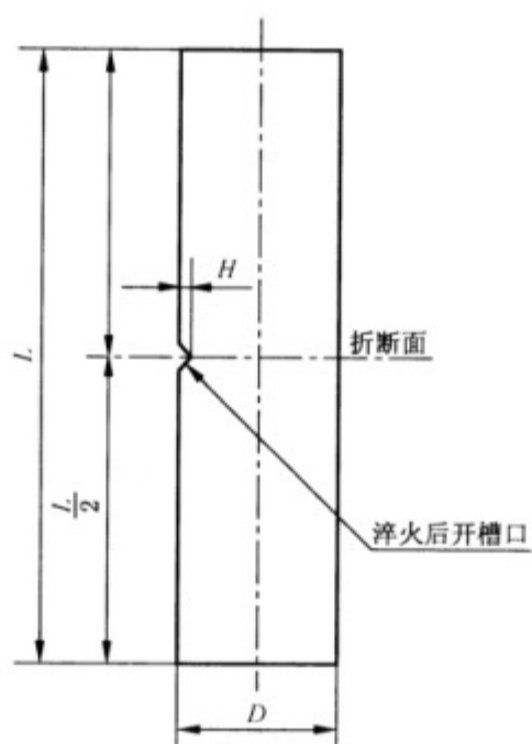
图 B.1 试样示意图
